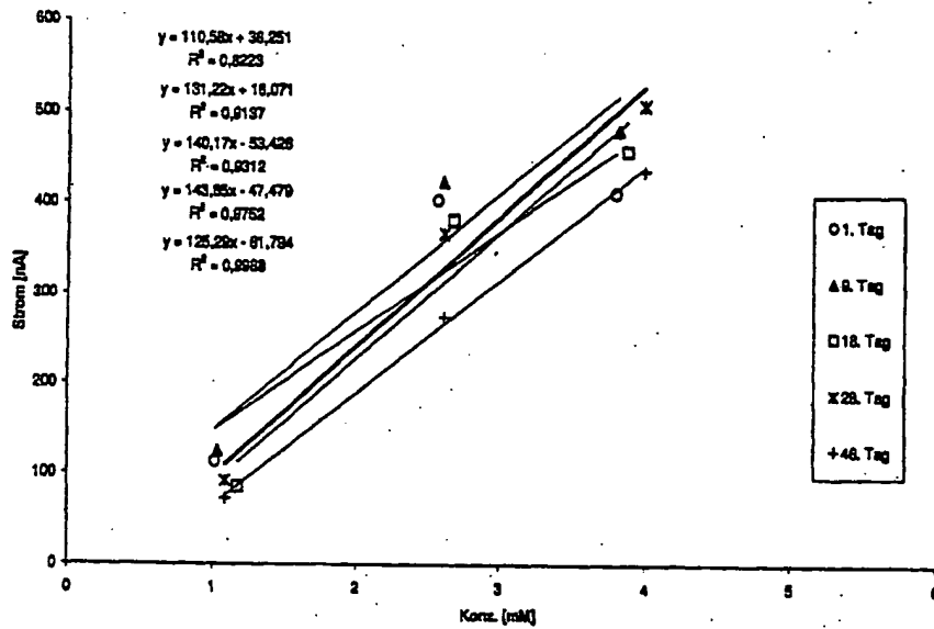
Abbildung 17: Sensitivität von TMPD-modifizierten Glukosebiosensoren mit Stärke-Schutzschicht in Abhängigkeit des Sensoralters
